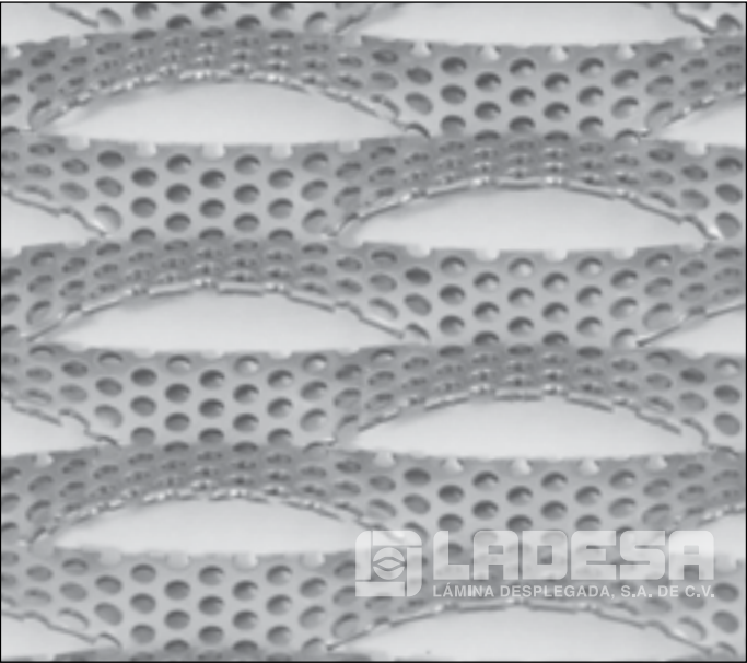
Louver 94 Perforado 39% área libre
